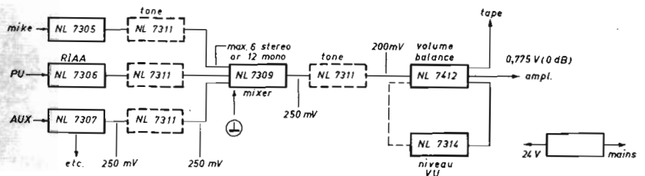
Voorbeeld van een combinatie van mengversterker-eenheden.
