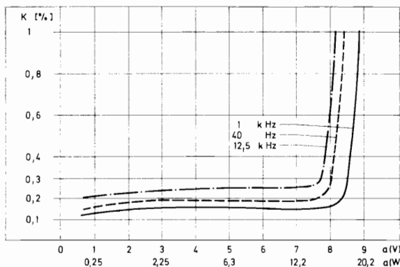
Fig. 3 Klirrfaktor bei 40 Hz, 1000 Hz, 12500 Hz in Abhängigkeit von der Ausgangsleistung.
