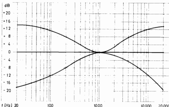
Fig. 5 Wirkungsweise der Klangregler. 0 dB = Baß- und Höhenregler in Mittenstellung.
