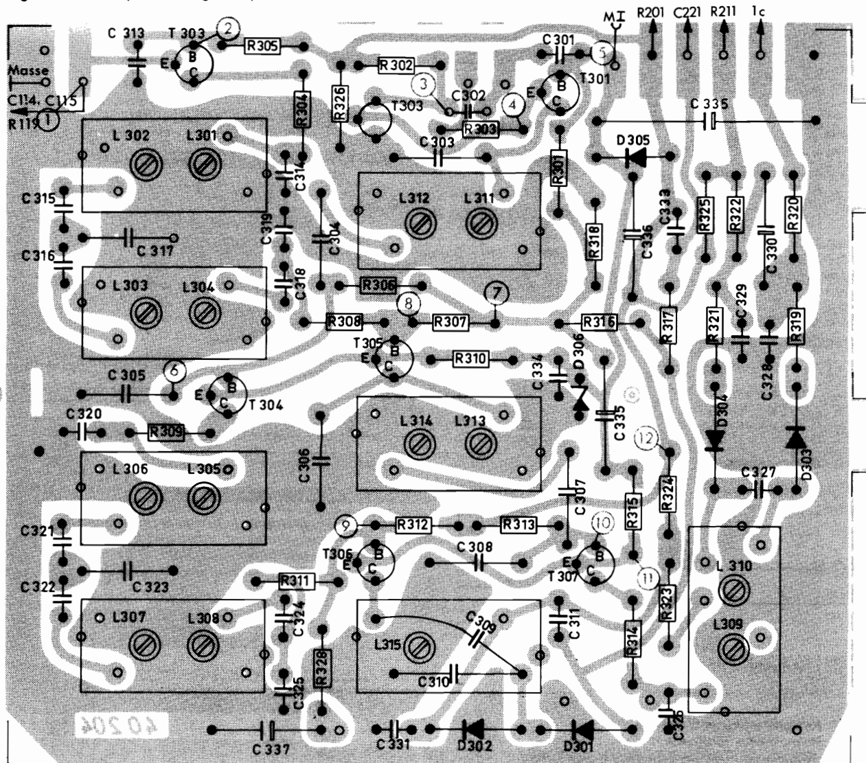
Fig. 6 ZF-Platte (Bestückungsseite)
