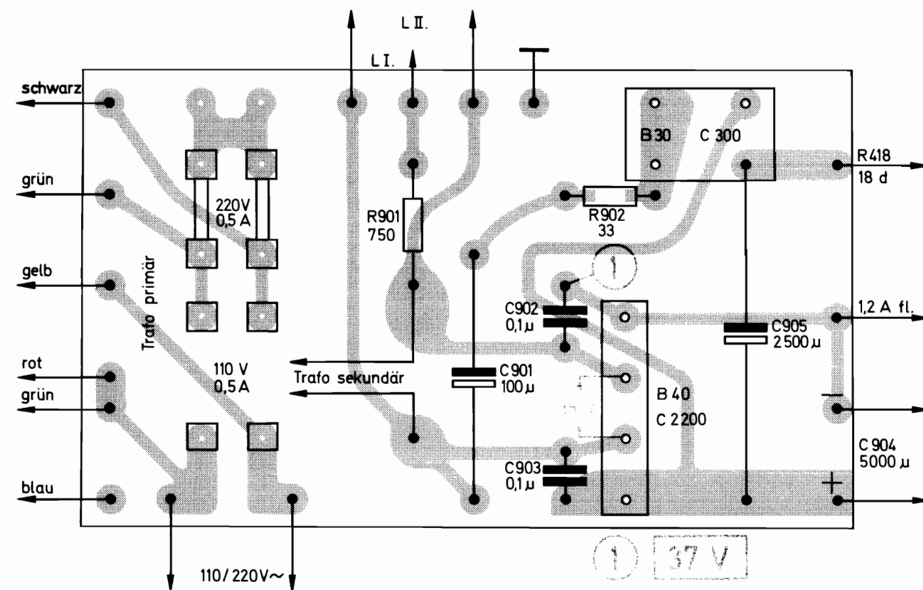
Fig. 15 Netzteil-Platte (Bestückungsseite)
