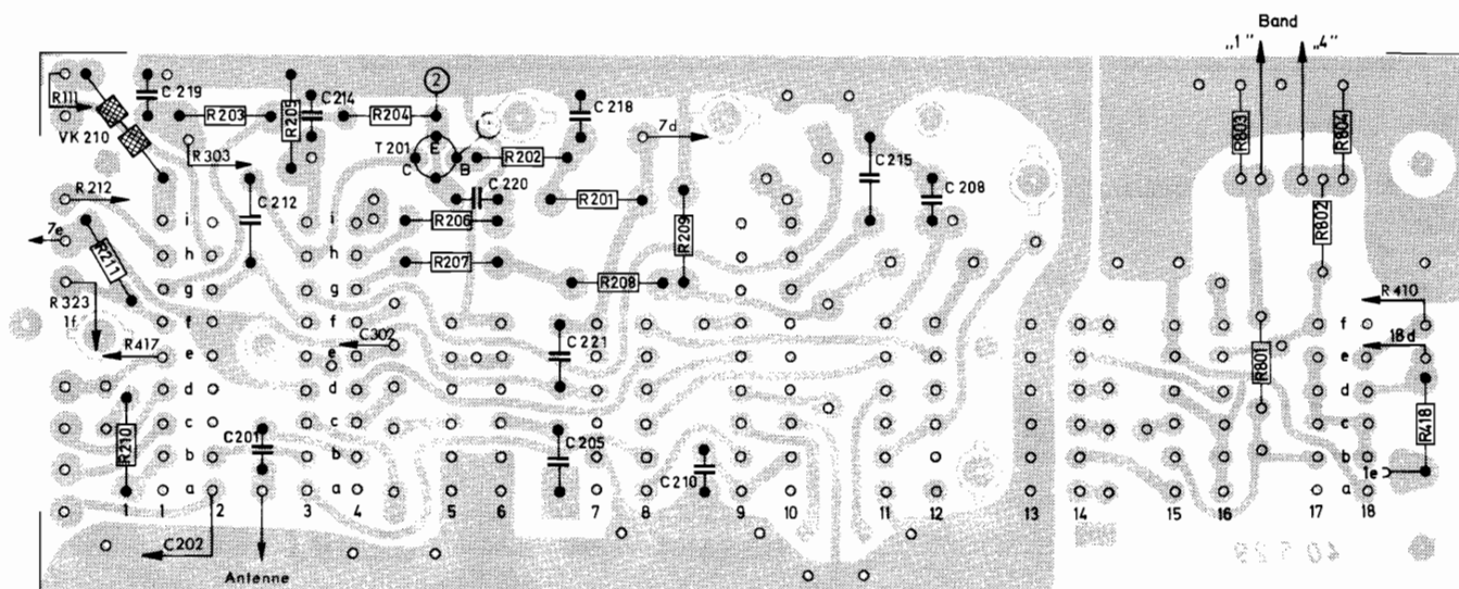
Fig. 10 Tastenschalter-Platte (Bestückungsseite)
