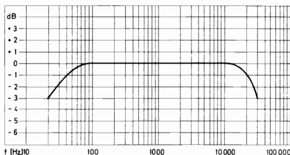
Fig. 2 Leistungsbandbreite gemessen nach DIN 45 500: 20 Hz bis 30 kHz.
