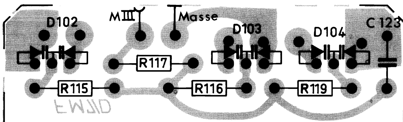
Fig. 8 Dioden-Platte (Bestückungsseite)
