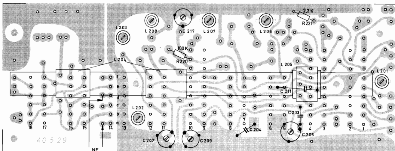
Fig. 9 Tastenschalter-Platte (Leiterseite)
