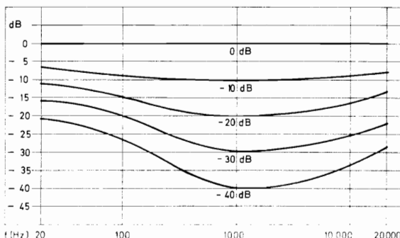
Fig. 4 Wirkungsweise der physiologischen Lautstärkeregelung. 0 dB = Lautstärkeregler offen.
