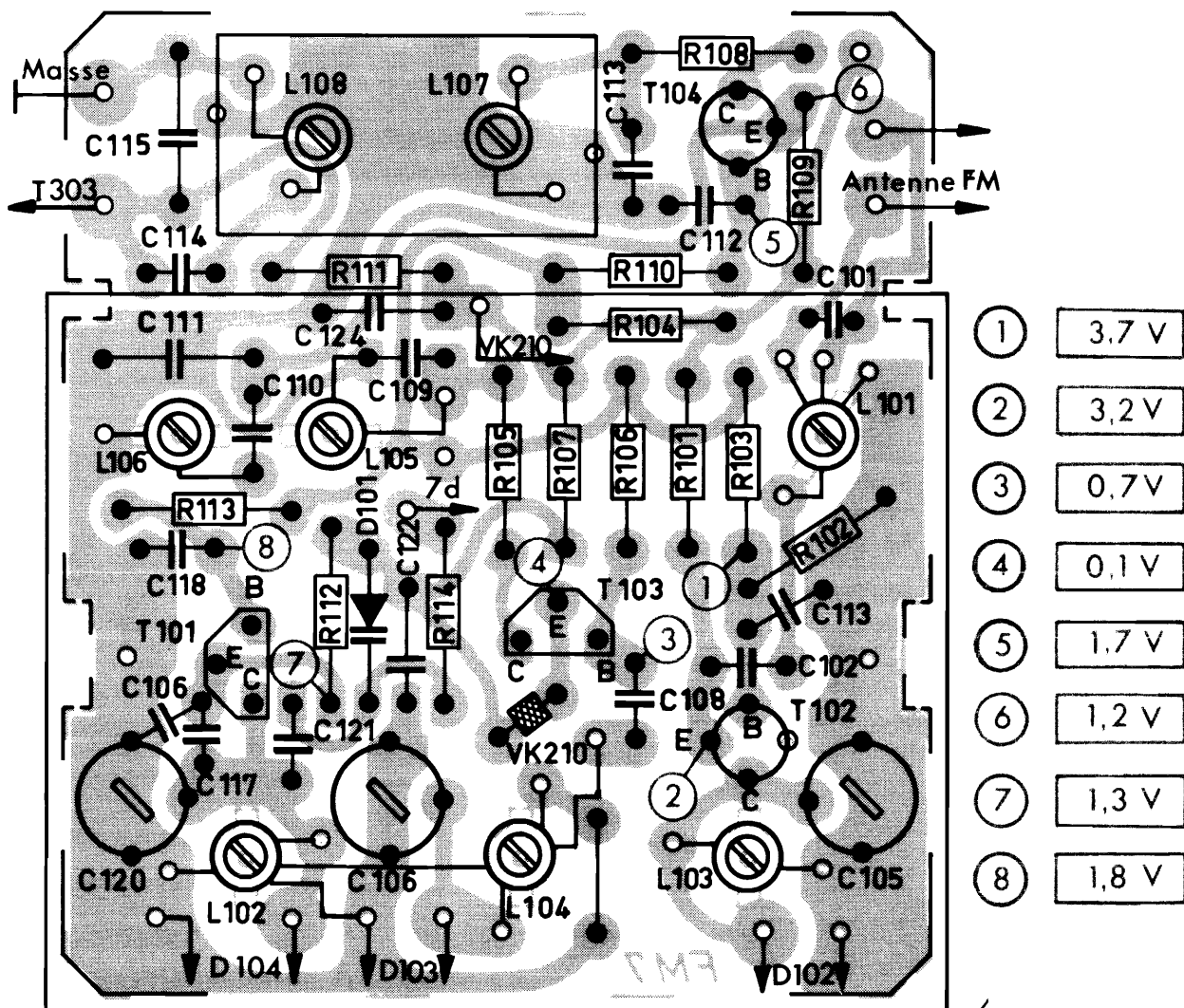
Fig. 7 UKW-Platte (Bestückungsseite)
