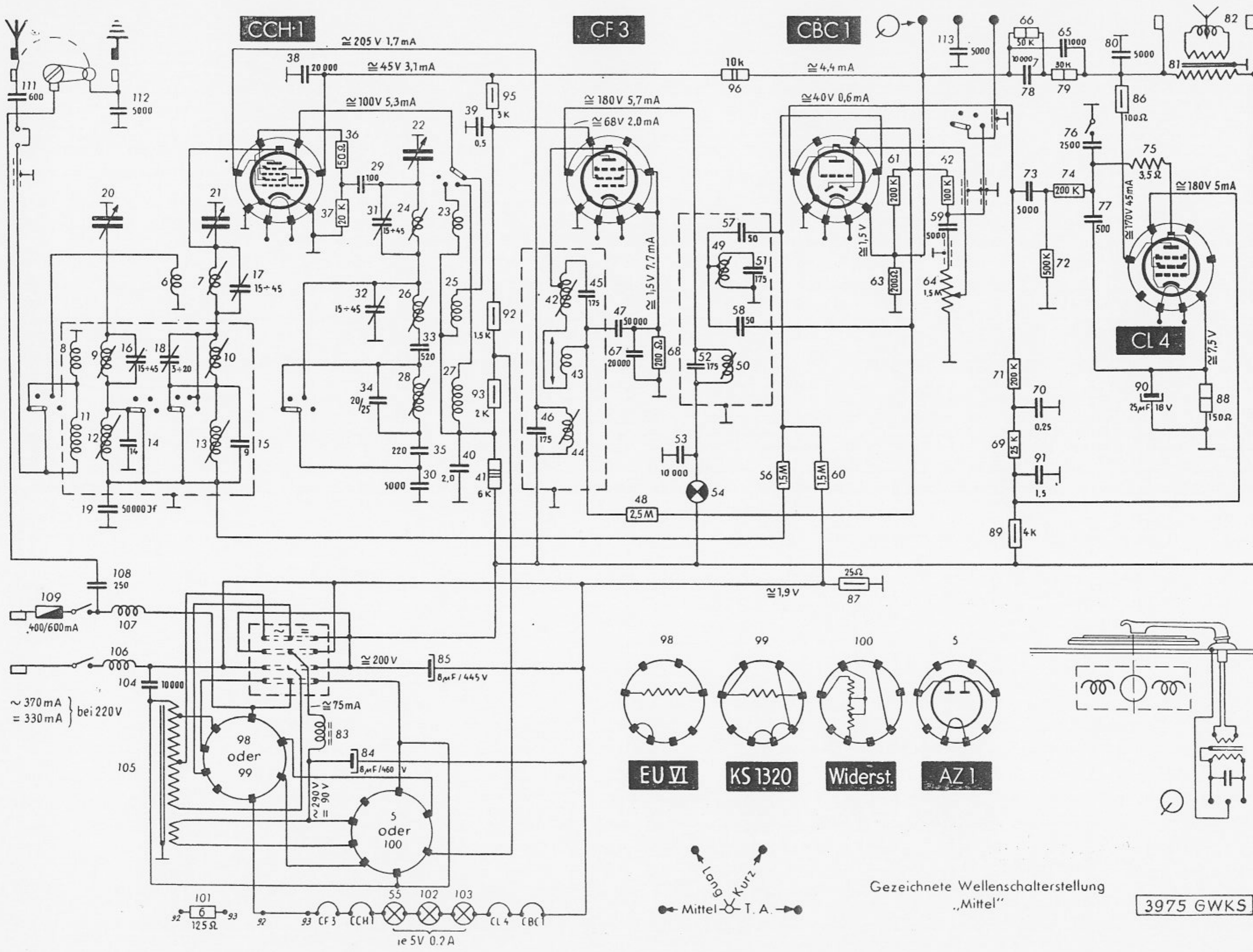
Schaltbild
