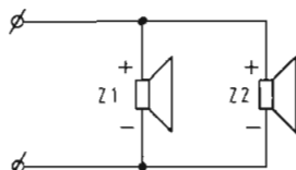
Afb. 4: Parallelschakeling. De impedantie volgt uit
