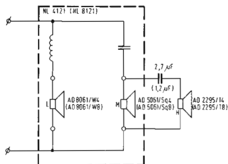
Afb. 2.: Eenvoudige driewegcombinatie.
