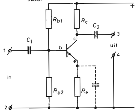
Afb. 9. Schakeling met tegenkoppeling via de emitterweerstand.
