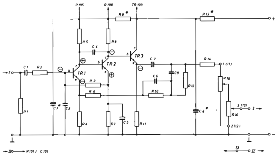
Afb. 12. Voorversterker van NL 7306.
