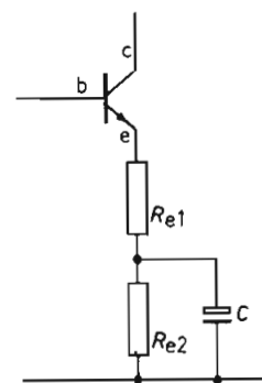
Afb. 10. Tegenkoppeling met „opgedeelde” emitterweerstand.
