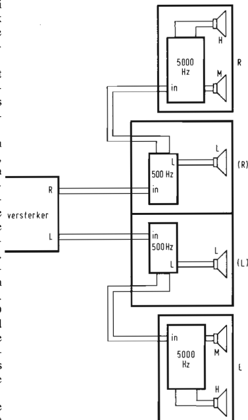
Afb. 3: Opstelling bij gemeenschappelijke wooferkast.
