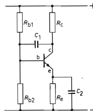
Afb. 11. Frequentie-afhankelijke tegenkoppeling.
