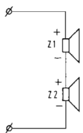
Afb. 3: Serieschakeling van luidsprekers. De impedantie (Z) wordt berekend uit Z_{tot} = Z_1 + Z_2 + \dots + Z_n
