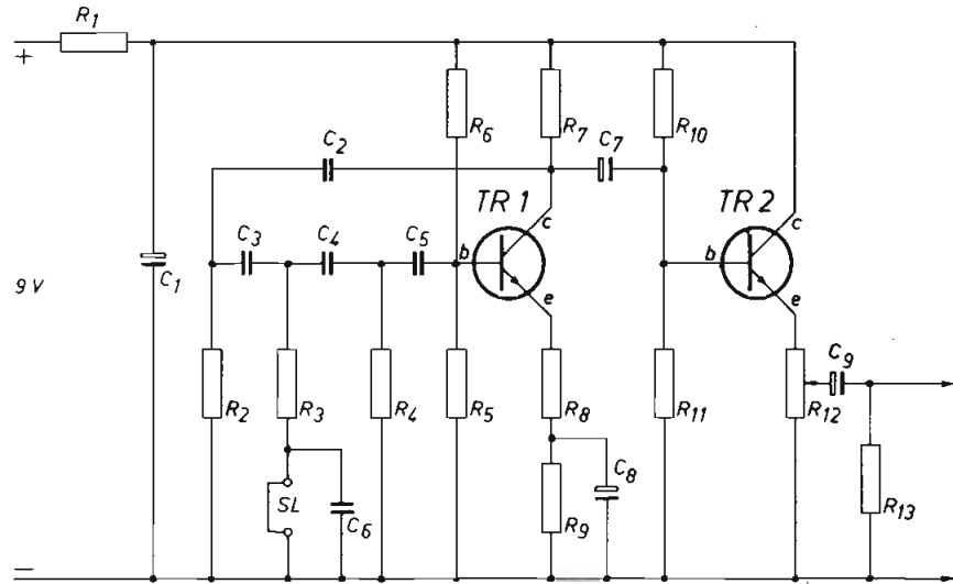
Afb. 14. Schema van de 1000 Hz-generator R 6830.
