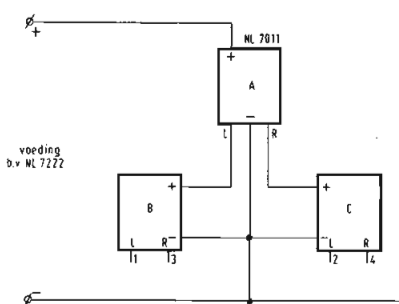
De schakeling met drie onderdelenpakketten NL 7011
