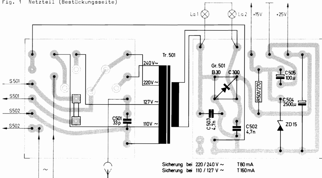
Fig. 1 Netzteil (Bestückungsseite)
