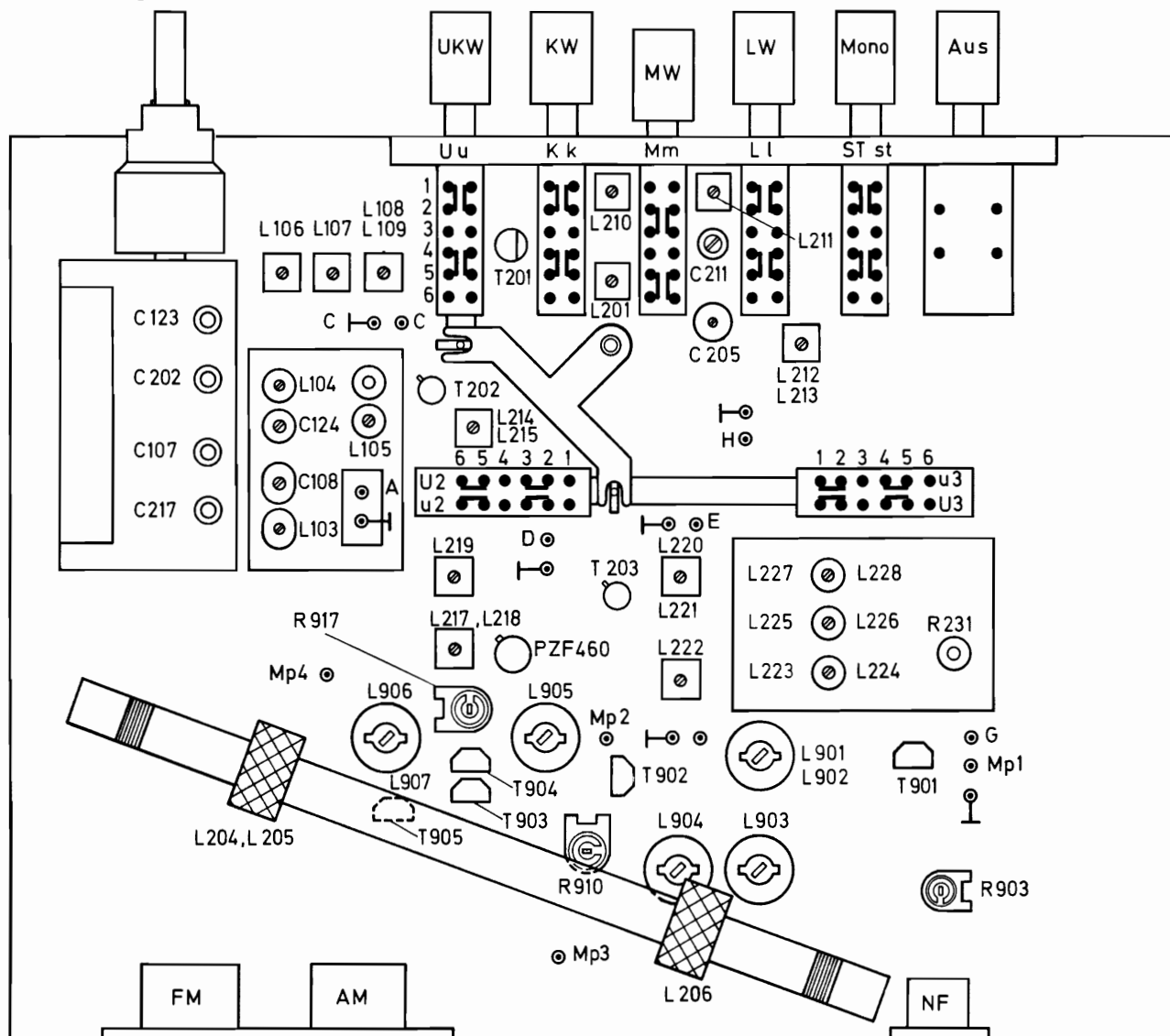
Fig. 4 Abgleichpunkte
