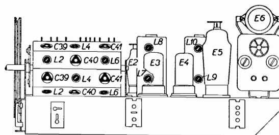
Sladovací prvky
